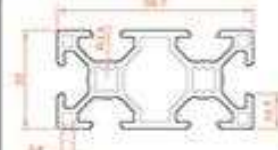
نقشه ۳۰x۶۰
